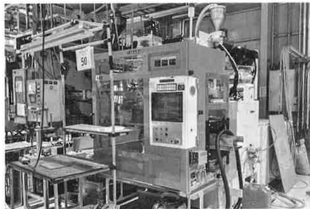
新規導入した電動ブロー成形機
